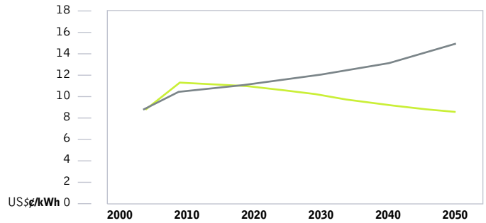
figura 6.8: Argentina: desarrollo de los costos de generación de electricidad bajo los dos escenarios
