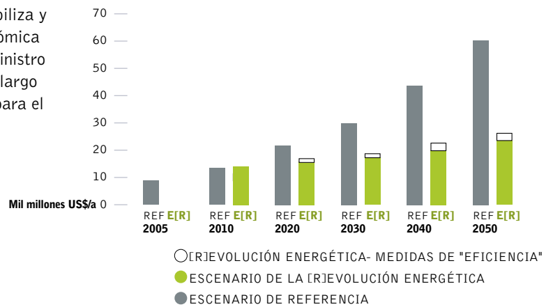
figura 6.9: Argentina: desarrollo de costos de suministro de electricidad total
