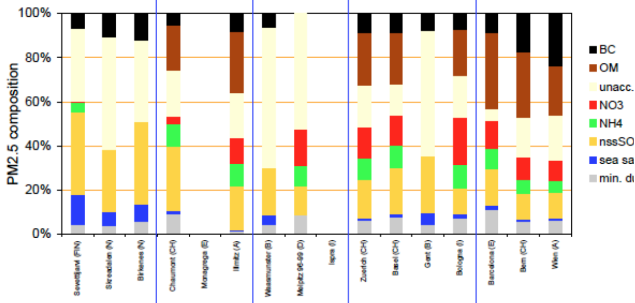
Appendice 3. Composizione del PM10 e del PM2.5 in 16 città europee.
