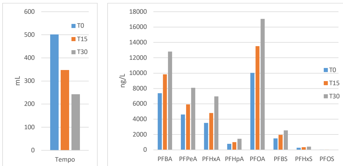
Figura 3 Variazione del volume (mL) dell'acqua di pozzo e della concentrazione di PFAS (ng/L) nella stessa acqua durante l'ebollizione (T0 inizio, T15 dopo 15 minuti e T30 dopo 30 minuti).
